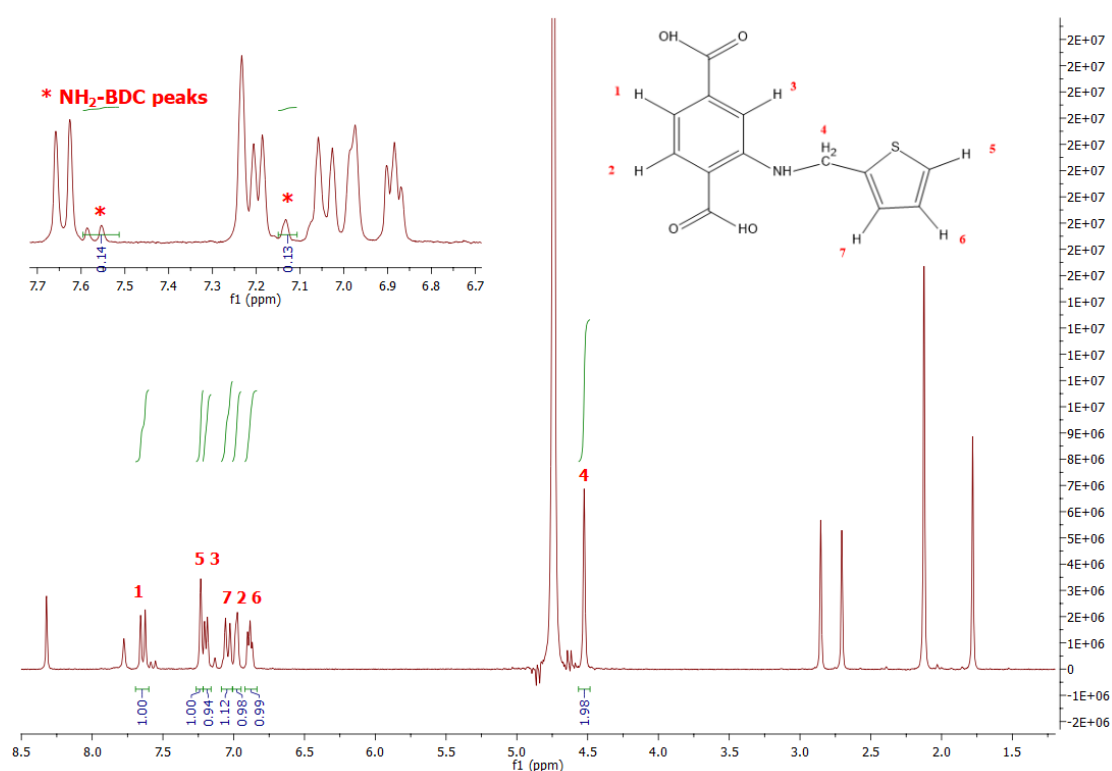
Εικόνα 3.22: Φάσμα ^1\text{H-NMR} του MOR-3 as synthesized. Ένθετο: Επισήμανση της ολοκλήρωσης των πρωτονίων του \text{NH}_2\text{-BDC}^{2-} που προκύπτει από τη διάσπαση του \text{TATP}^{2-} .
