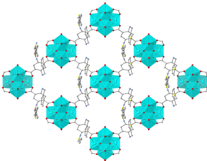
Εικόνα 3.19: Απεικόνιση του MOR-3 σε επίπεδο κάθετο στον άξονα b. Στη απεικόνιση δεν εμφανίζονται τα άτομα υδρογόνου για λόγους ευκρίνειας.
