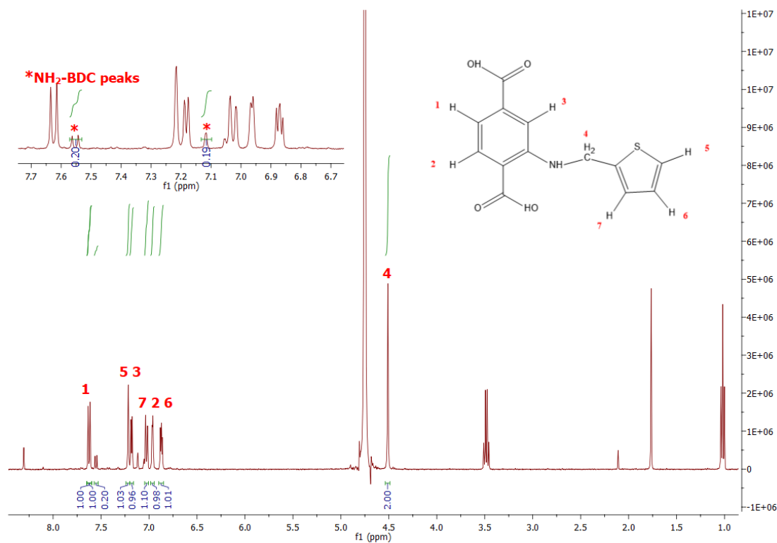
Εικόνα 3.23: Φάσμα 1 H-NMR του MOR-3 μετά την ανταλλαγή διαλυτών με αιθανόλη. Ένθετο: Επισήμανση της ολοκλήρωσης των πρωτονίων του NH 2 -BDC 2- που προκύπτει από τη διάσπαση του TATP 2- .
