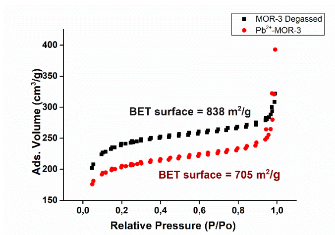
Εικόνα 3.38: Ισόθερμοι ρόφησης-εκρόφησης N_2 για το MOR-3 πριν και μετά από τη ρόφηση Pb^{2+} .
